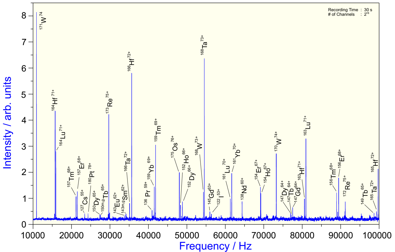
Schottky Spectrum
